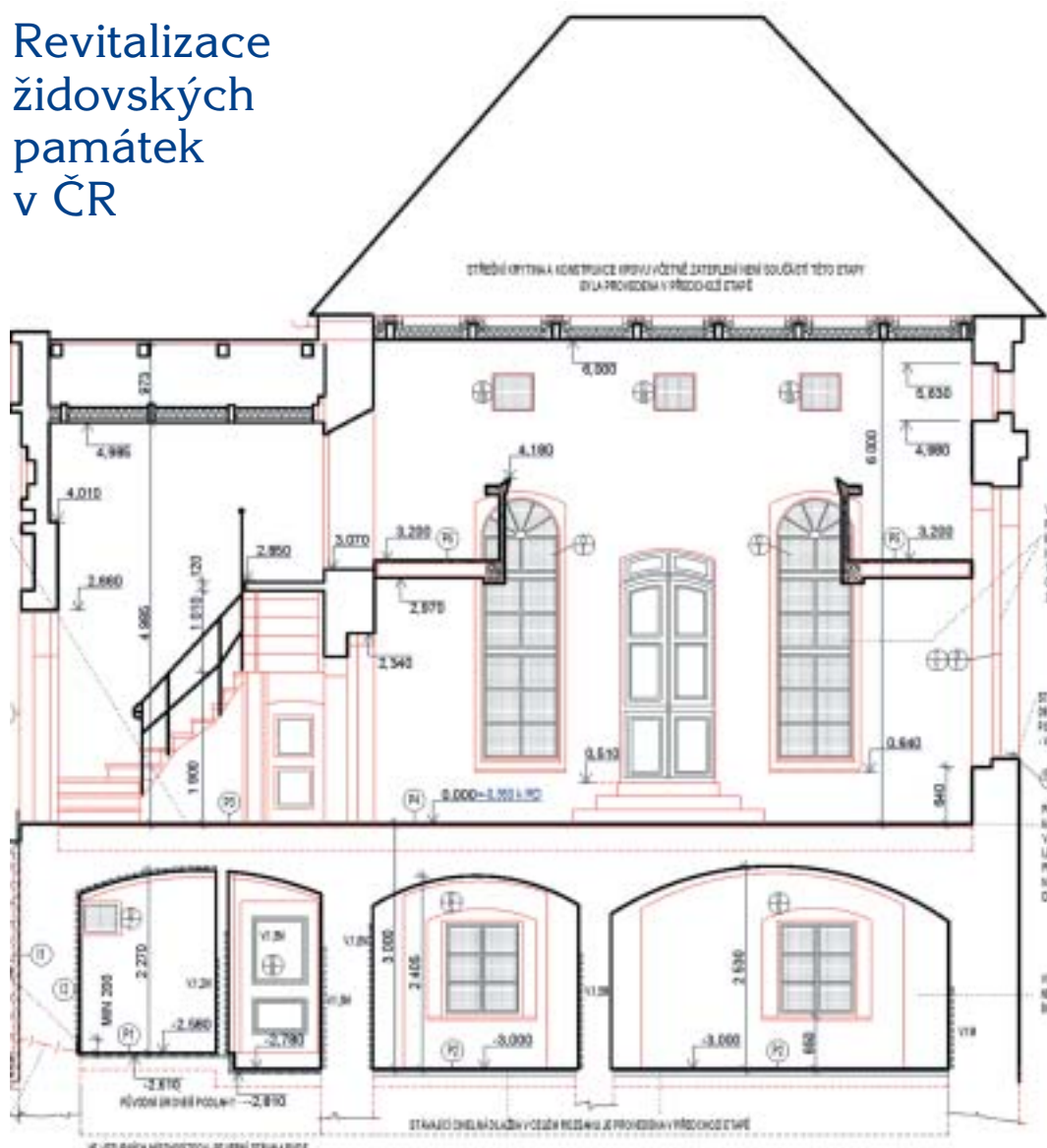
Synagoga v Ústěku – příčný řez.
